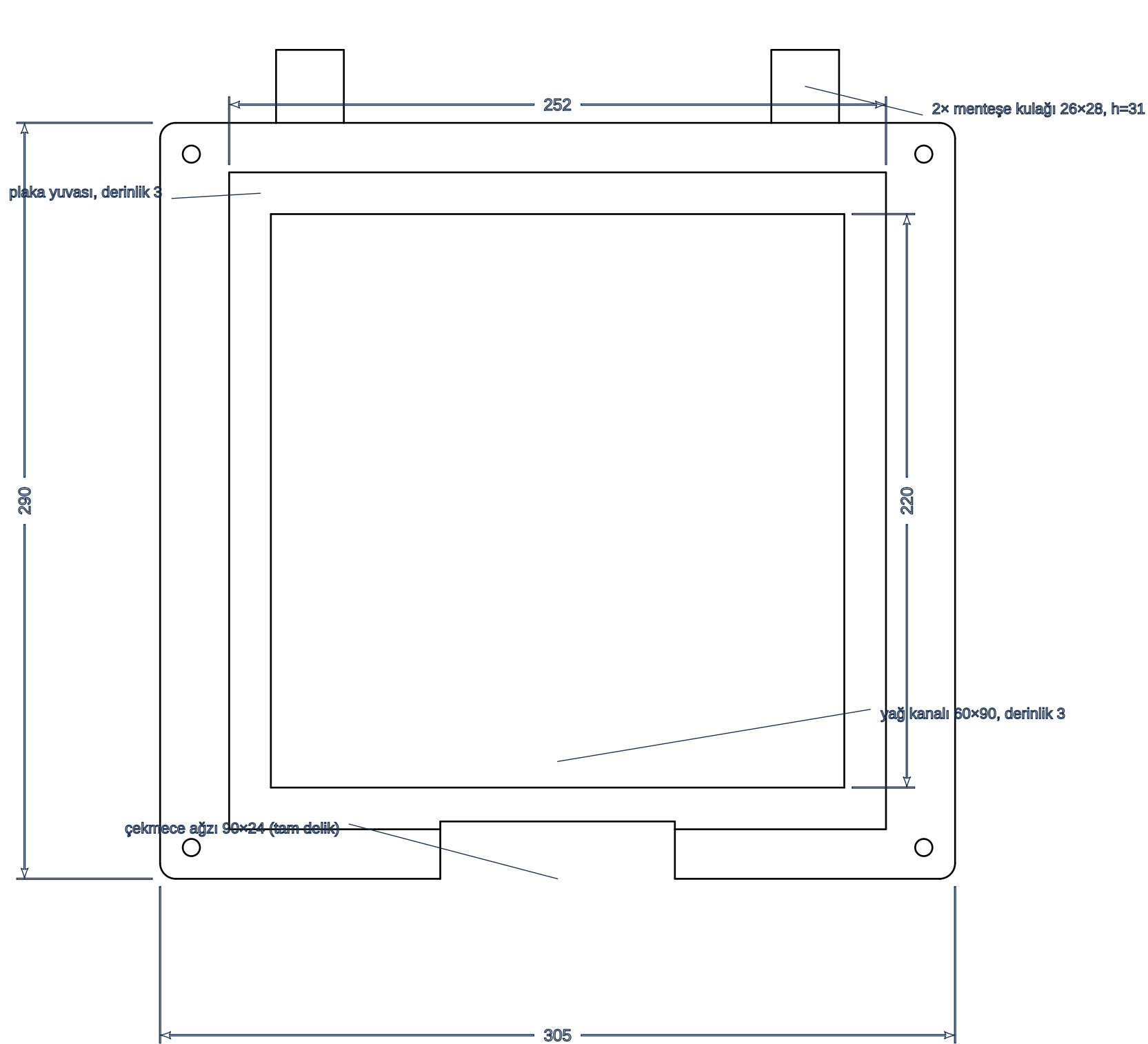
ALT TAŞIYICI — KATMAN 3
